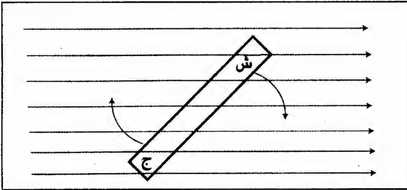
الشكل (38): تأثير حقل مغناطيسي متجانس على ثنائي قطب هو خلق قوة فتل تجعله يدور بحيث يكون القطب الشمالي للمغناطيس مصطفا مع خطوط الحقل.
